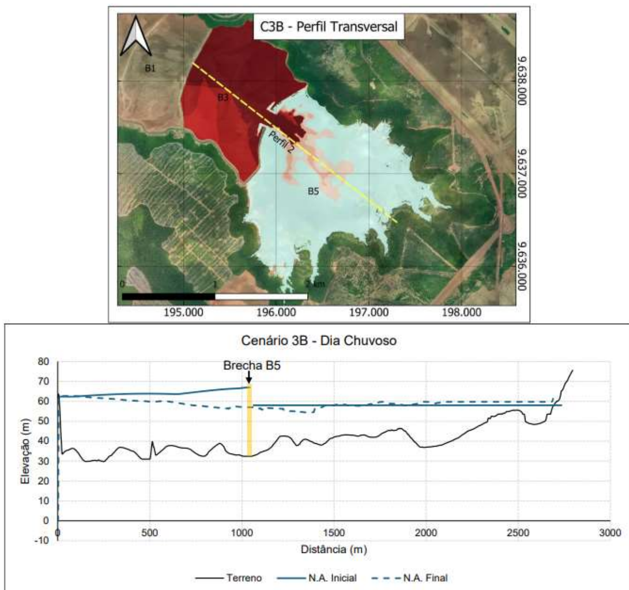
Figura 9-4 - Perfil Transversal – Cenário 3B
